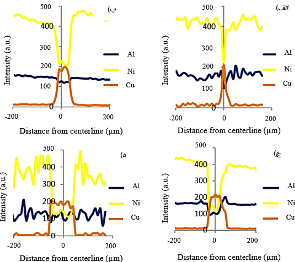
شکل ۴- ارزیابی خطی عنصری اتصال با لایه میانی مس در زمان‌های: الف) ۳۰، ب) ۶۰، ج) ۹۰ و د) ۱۲۰ دقیقه
