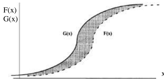
شکل (۱) توابع توزیع تجمعی فرصت سرمایه‌گذاری F و G [۱۷]
