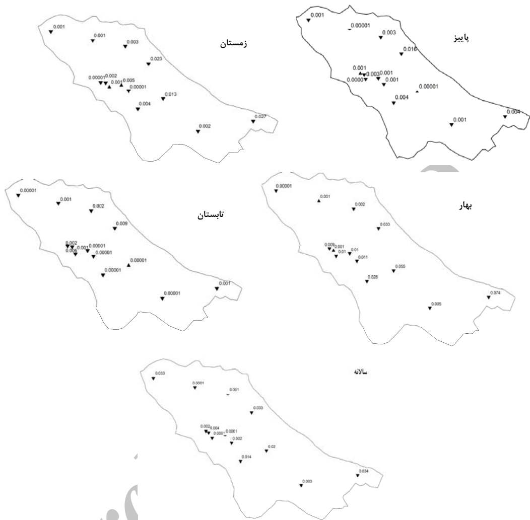
شکل ۷: بزرگی روند سالانه و فصلی دبی در ایستگاه‌های مورد مطالعه در حوزه‌ی آبخیز کشف‌رود (مثلت روبه بالا مقدار مثبت و روبه پایین مقدار منفی را نشان می‌دهد)
