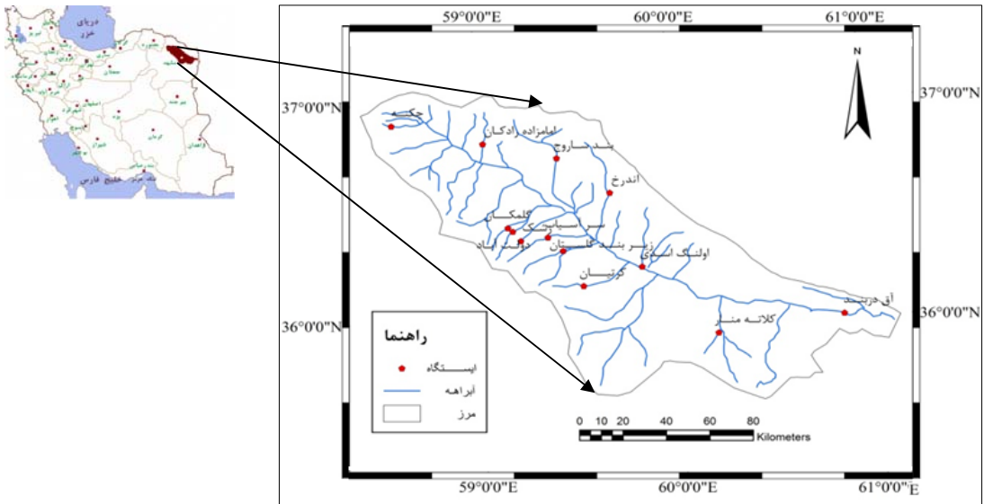
شکل ۱: موقعیت حوزه آبخیز کشفرود در ایران و موقعیت ایستگاه‌های هواشناسی و هیدرومتری در سطح حوزه آبخیز کشفرود مأخذ: نگارندگان
