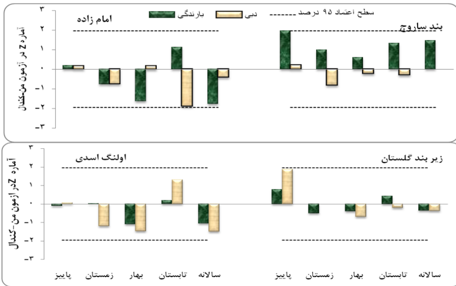
شکل ۵: روند در ایستگاه‌های امامزاده، کرتیکان، اندروخ و چکنه علیا مأخذ: نگارندگان
