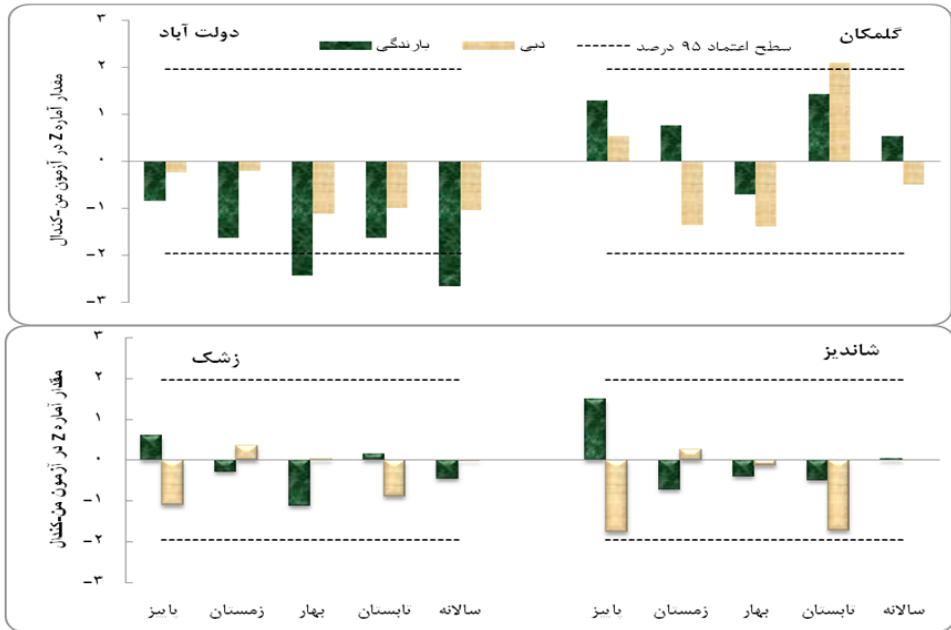
شکل ۲: آماره Z آزمون من-کندال در ایستگاه‌های گلمکان، دولت‌آباد، زشک و شان‌دیز مأخذ: نگارندگان
