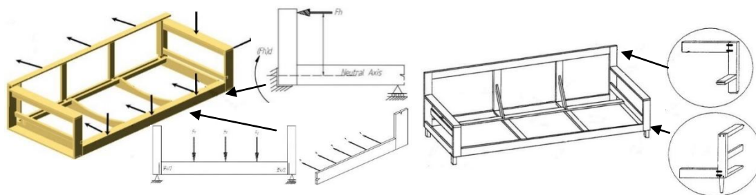
شکل ۱- اتصال گوشه ای L و T اسکلت مبلمان راحتی سه نفره زیر نیروهای وارده [۳]
