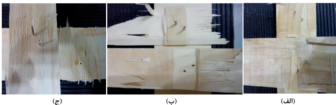
شکل ۹- نمونه‌هایی از شکست اعضای اتصالات‌های ساخته‌شده با چسب الف (OSL ب) تخته چندلا ج) چوب صنوبر
