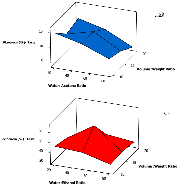
شکل ۳- نمودار سطح پاسخ اثر نسبت حلال به زعفران و آب به حلال (الف- استن و ب- اتانل) بر مقدار طعم زعفران (پیکروکروسین)
