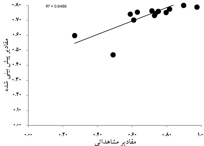
نمودار ۲: نمودار پراکنش برای مقادیر مشاهده و پیش بینی شده با استفاده از روش شبکه عصبی (یافته‌های پژوهش)
