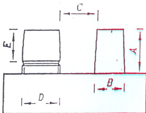
شکل ۵. ابعاد اندازه‌گیری
