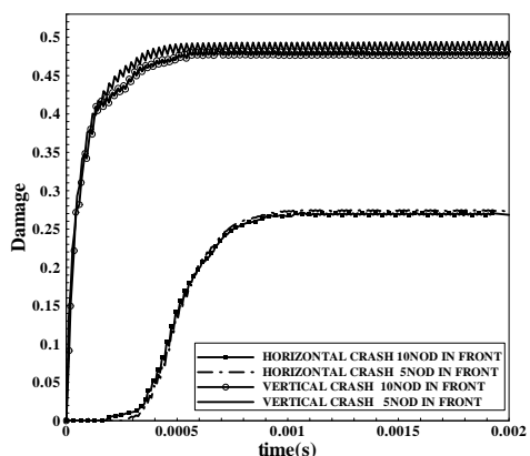
شکل ۳۴ مقایسهی رشد آسیب برای امتدادهای مختلف تصادم در فشار کاری در ناحیهی خارجی جداری مخزن
