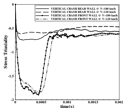
شکل ۲۳ تاریخچه‌ی تنش سه‌محوره برای نقطه‌ای در نواحی آسیب‌دیده‌ی تصادم عمودی در فشار کاری مخزن و سرعت‌های متفاوت
