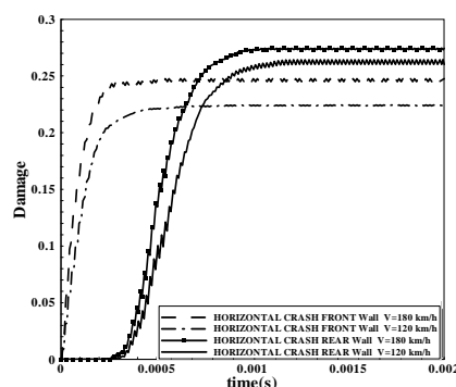
شکل ۱۰ رشد آسیب برای نقطه‌ای در ناحیه‌ی آسیب‌دیده‌ی تصادم افقی در فشارکاری مخزن و سرعت‌های متفاوت
