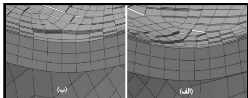
شکل ۲۵ نواحی زوال یافته در تصادم عمودی برای فشار ۲۰۰ bar و سرعت ۱۲۰ km/h، الف-عدسی مقابل مخزن، ب-عدسی پشت مخزن
