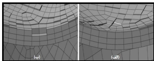
شکل ۲۷ نواحی زوال یافته در تصادم عمودی برای فشار ۵۰ bar و سرعت ۱۲۰ km/h، الف-عدسی مقابل مخزن، ب-عدسی پشت مخزن
