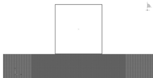
شکل ۲ مدل اجزا محدود برخورد پرتابه با دماغه تخت به صفحه‌ی هدف
