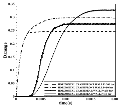
شکل ۱۱ رشد آسیب برای نقطه‌ای در ناحیه‌ی آسیب‌دیده‌ی تصادم افقی در سرعت ۱۸۰ km/h و فشارهای متفاوت مخزن
