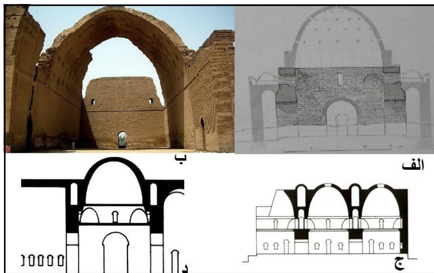
تصویر ۹. طاق با چفد هلوچین و کنوبندی در بناهای ساسانی: الف) طاق با چفد هلوچین در چهارقاپو قصرشیرین (روتز، ۱۳۸۷: ۶۹۳). ب) طاق با چفد هلوچین در کاخ خسرو در تیسفون ( https://www.kojaro.com ). ج) کنوبندی در پیرامون گنبد کاخ اردشیر در فیروزآباد (هوگی، ۱۳۷۹: ۸۱). د) کنوبندی در پیرامون گنبد در کاخ-قلعه اردشیر (قلعه‌دختر) در فیروزآباد (هوگی، ۱۳۷۹: ۵۵). ◀
