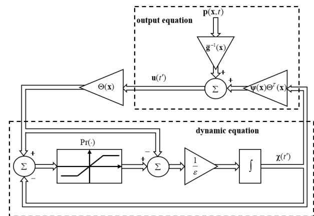
شکل ۱- ساختار داخلی شبکه عصبی بازگشتی تصویر (PRNN)
