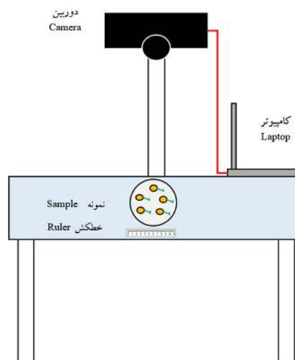
شکل ۱- سامانه دریافت تصویر دیجیتال از نمونه و پردازش آن Figure 1- Digital Imaging system for image acquisition from samples and further analysis
