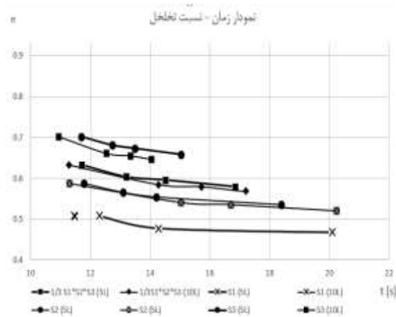
شکل ۱۱- زمان- نسبت تخلخل در ماسه ها
