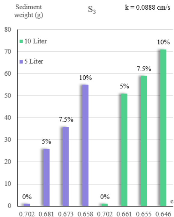
شکل ۹- وزن رسوب- نسبت تخلخل در سری ماسه یک سانتی متری
