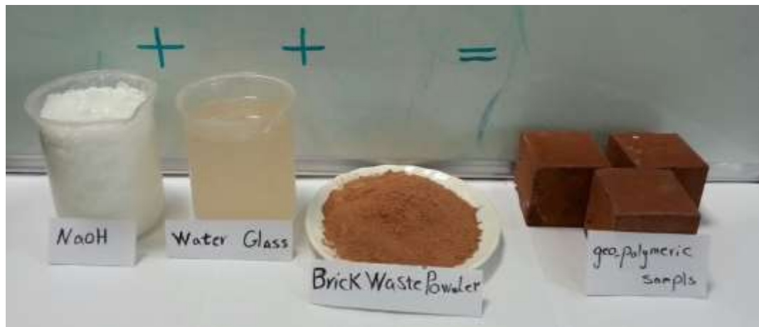
Fig. 3. Cubic geopolymeric 50×50×50-mm samples
