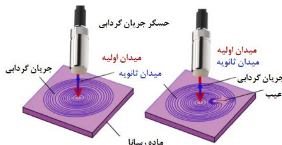
شکل ۵) اصول آزمون جریان گردابی [۱۸]
