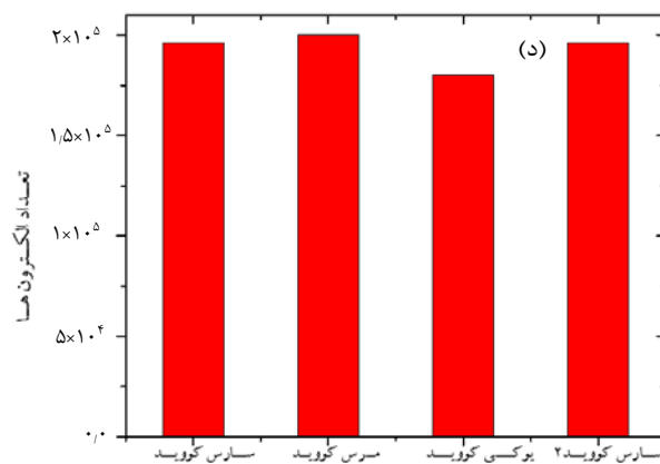
شکل ۶. الف) تعداد زنجیره‌های پروتئینی، ب) تعداد اتم‌ها، ج) تعداد پیوندها و د) تعداد الکترون‌های موجود در اسپایک‌های مورد بررسی در این تحقیق را نشان می‌دهد.
