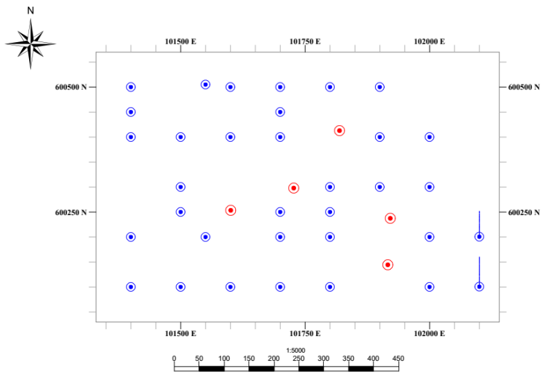
شکل ۱۱- موقعیت گمانه‌های پیشنهادی نسبت به گمانه‌های اولیه (دید از بالا)
