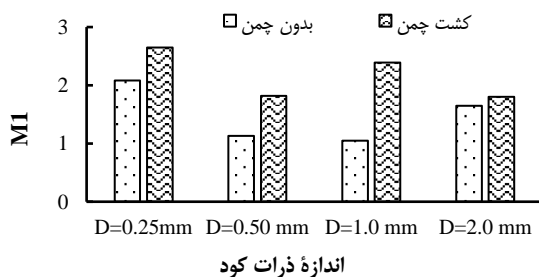
شکل ۱۱- مقادیر گشتاور مرتبه اول در تیمارها
