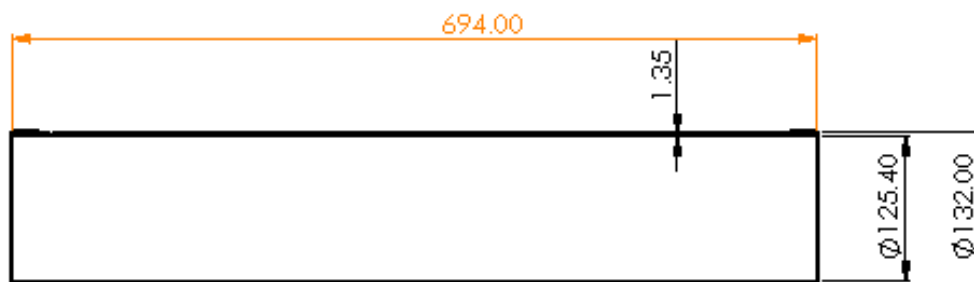
شکل ۴ ابعاد نهایی نمونه فولاد D6ac بعد از فرایند فلوفرمینگ
