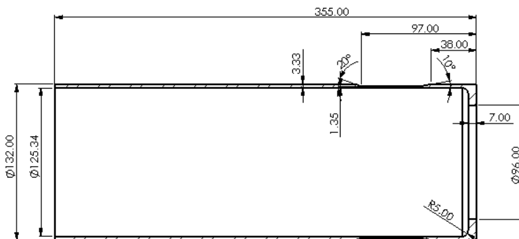
شکل ۳ ابعاد پریفرم فولاد D6ac جهت شروع فرایند فلوفرمینگ (بر حسب میلیمتر)
