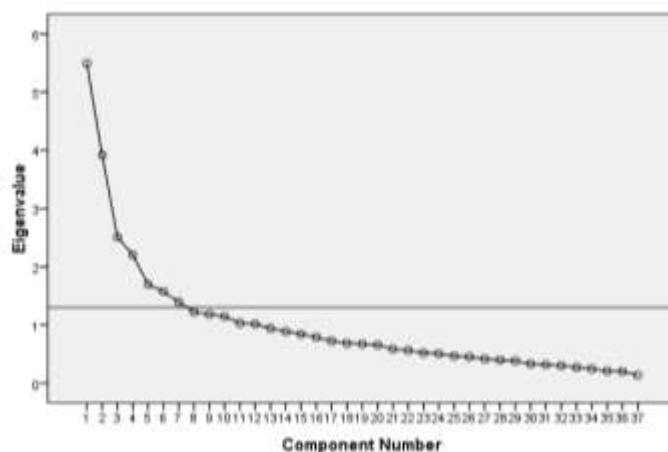
شکل ۲. نمودار سنگریزه و خط افقی تعیین عامل (با مقدار ویژه بزرگ‌تر از ۱,۳)
