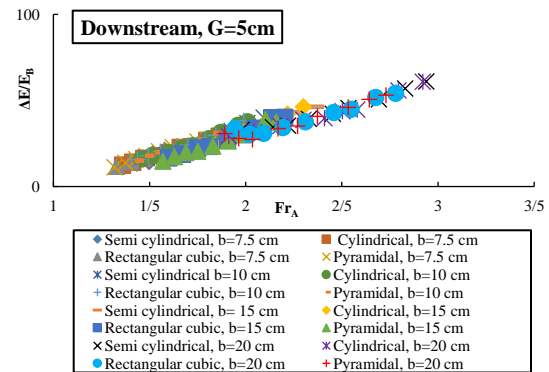
شکل ۷- تغییرات استهلاک انرژی با آستانه در هندسه‌های مختلف در حالت مماس بر پایین دست دریچه.
