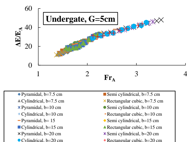
شکل ۹- تغییرات استهلاك انرژی با هندسه‌های مختلف آستانه در حالت آستانه زیر دریچه کشویی.
