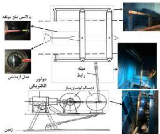
شکل ۱- مدل و تجهیزات تست
