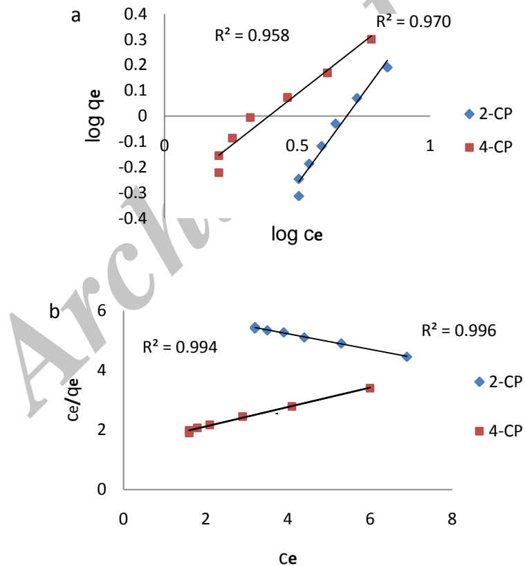
Fig6. Isotherm models: (a) Freundlich (b) Langmuir
