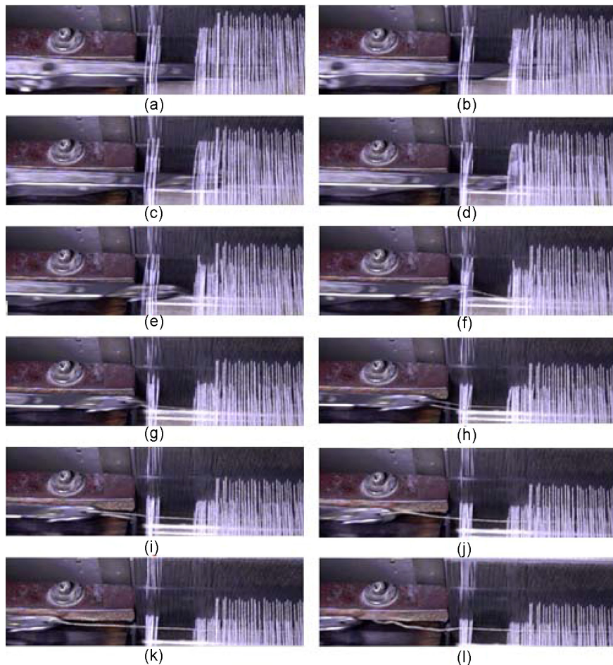
Fig. 2. Weft yarn exit in different times: (a) 0.001 s, (b) 0.002 s, (c) 0.003 s, (d) 0.004 s, (e) 0.005 s, (f) 0.006 s, (g) 0.007 s, (h) 0.008 s, (i) 0.009 s, (j) 0.01 s, (k) 0.011 s, and (l) 0.012 s.
