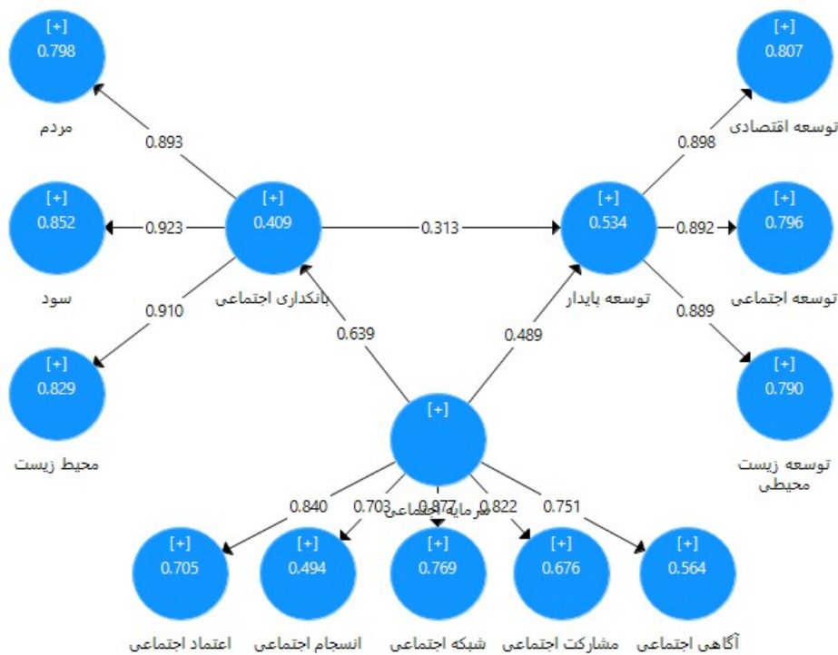
شکل ۵- ضرایب مسیر (ضرایب اثر یا رگرسیون) و ضرایب تبیین (ضرایب تعیین) در مدل ساختاری
