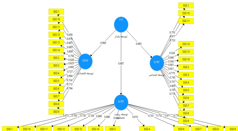
شکل ۳- بارهای عاملی در برآورد مدل اندازه‌گیری شاخص‌های توسعه پایدار
