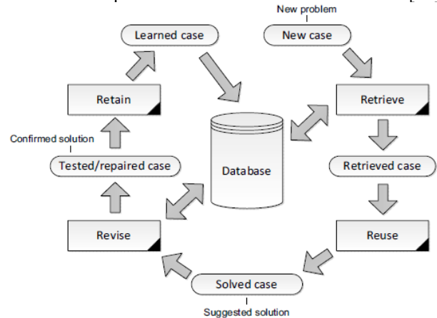
Fig. 3. CBR cycle[15].
