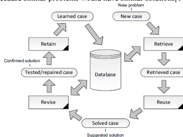
Fig. 3. CBR cycle[15].
