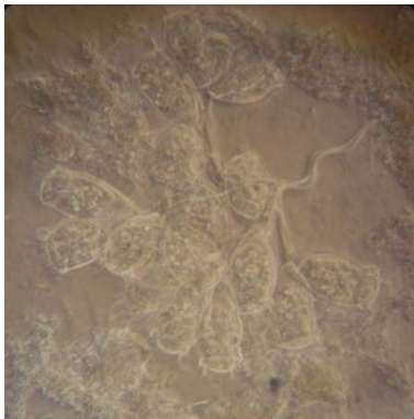
Vorticella
