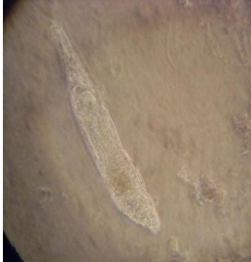
Rotifera
