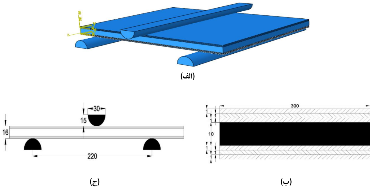
شکل ۱. هندسه مورد بررسی به همراه ابعاد الف) نمای کلی هندسه ب) نحوه قرارگیری رویه ها ج) ابعاد تکیه گاهها و نحوه قرارگیری آنها. (کلیه ابعاد بر حسب میلیمتر است)
