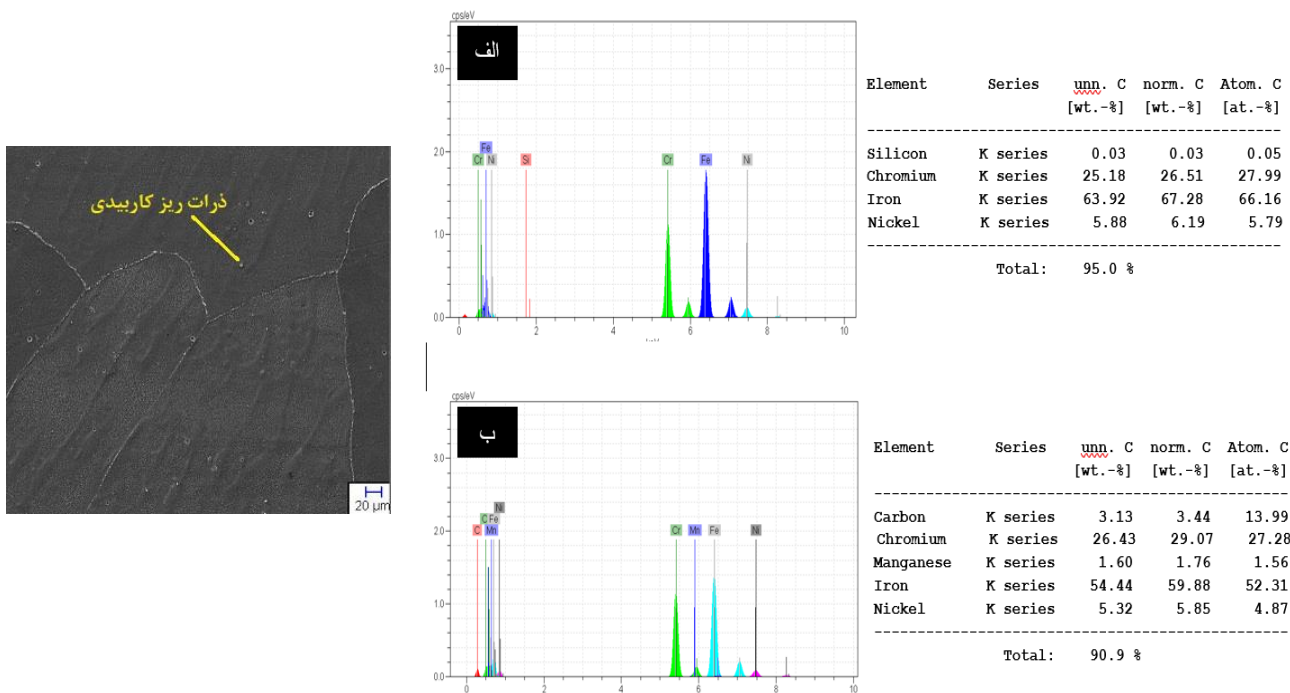
شکل ۶. تصویر میکروسکوپی الکترونی روبشی به همراه آنالیز طیف سنجی پراش انرژی پرتو ایکس لایه دوم روکش ER ۳۱۲ (الف) فاز زمینه، (ب) ذرات کاربیدی
