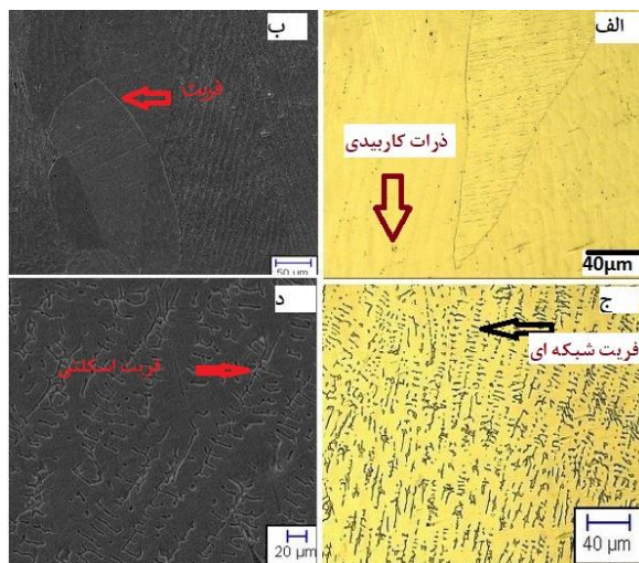
شکل ۷. تصاویر میکروسکوپی نوری و الکترونی (ER ۳۰۹: الف-ب) لایه اول روکش، ج-د) لایه دوم روکش
