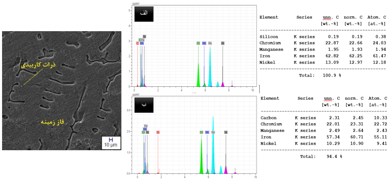
شکل ۹. تصویر میکروسکوپی الکترونی روبشی به همراه آنالیز طیف سنجی پراش انرژی پرتو ایکس لایه دوم روکش ۳۰۹ ER (الف) فاز زمینه، ب) ذرات کاربید
