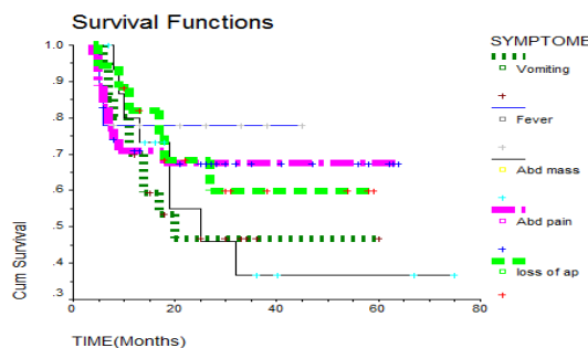
نمودار ۶: مدت بقا بر حسب علائم
