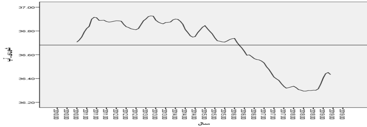
شکل ۴- روند شوری آب خلیج چابهار از سال ۲۰۱۰ تا ۲۰۱۹
