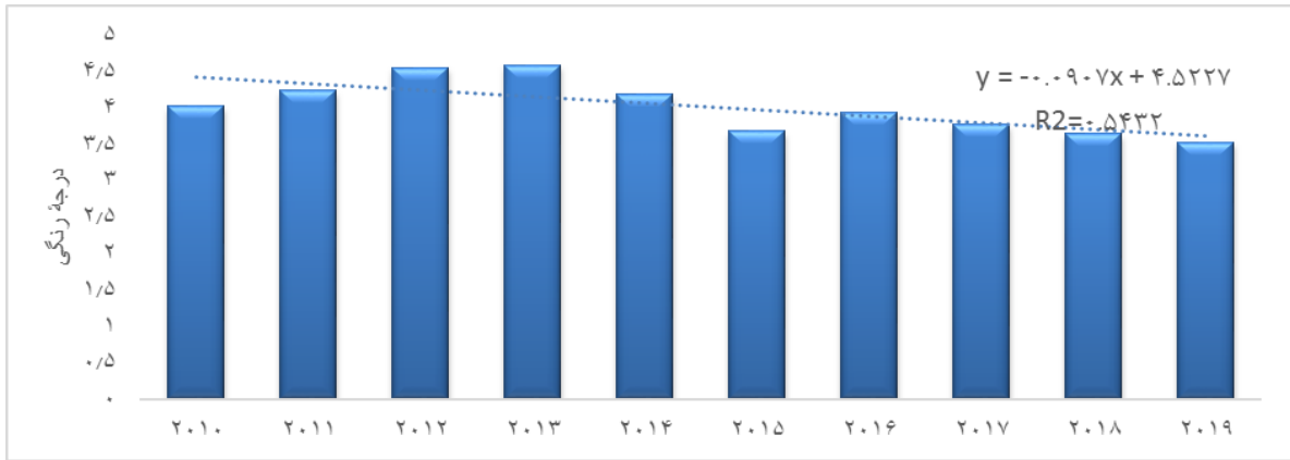
شکل ۱- نمودار وضعیت درجه رنگی شاخص سلامت مرجان‌های توده‌های خلیج چابهار از سال ۲۰۱۰ تا ۲۰۱۹
