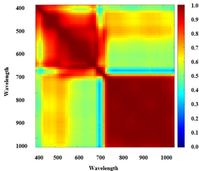
شکل ۲- میزان همبستگی بین طول موج‌ها در این مطالعه. همبستگی بالای ۹۵ درصد بین طول موج‌های فرورسرخ وجود دارد. Fig. 2. Pairwise correlation between the spectral bands. The near infrared bands were highly correlated (>95%).
