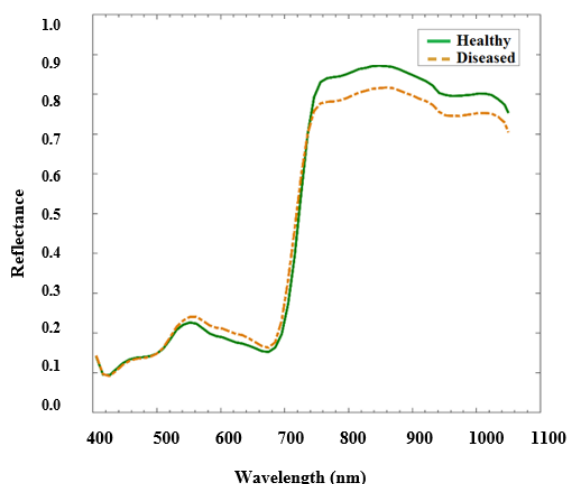
شکل ۳- میانگین بازتابش برگ‌های سالم و بیمار Fig. 3. The average of spectral reflectance for the healthy and diseased leaves
