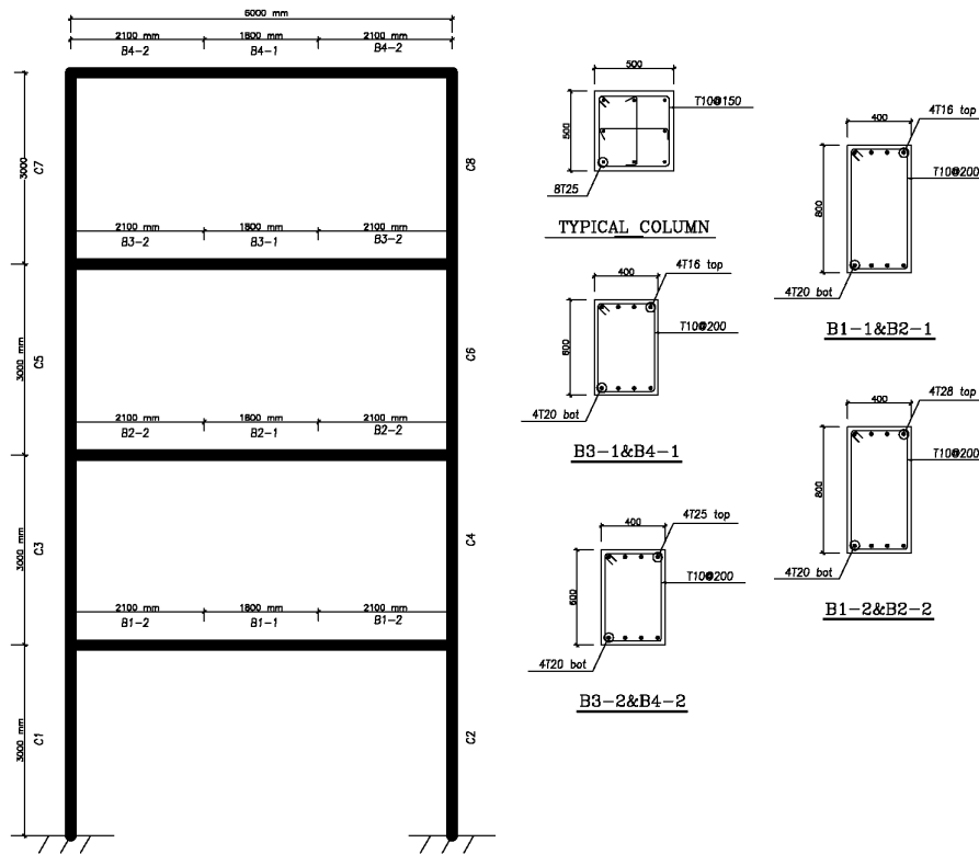
Frame Elevation
