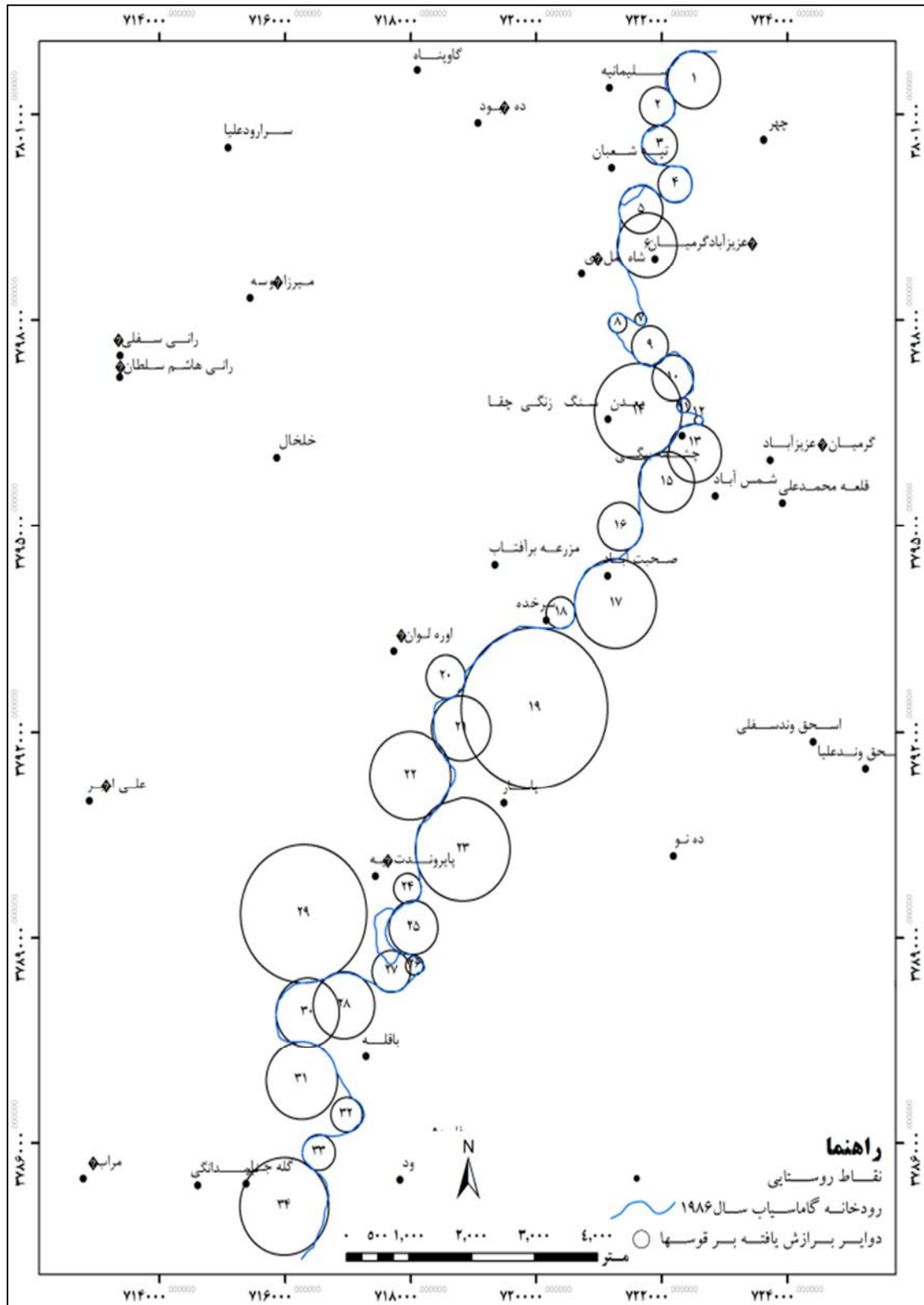
شکل ۲. دوایر برازش یافته با مآندرهاى رودخانه‌ی گاماسیاب در دشت بیستون الف) سال ۱۹۸۶
