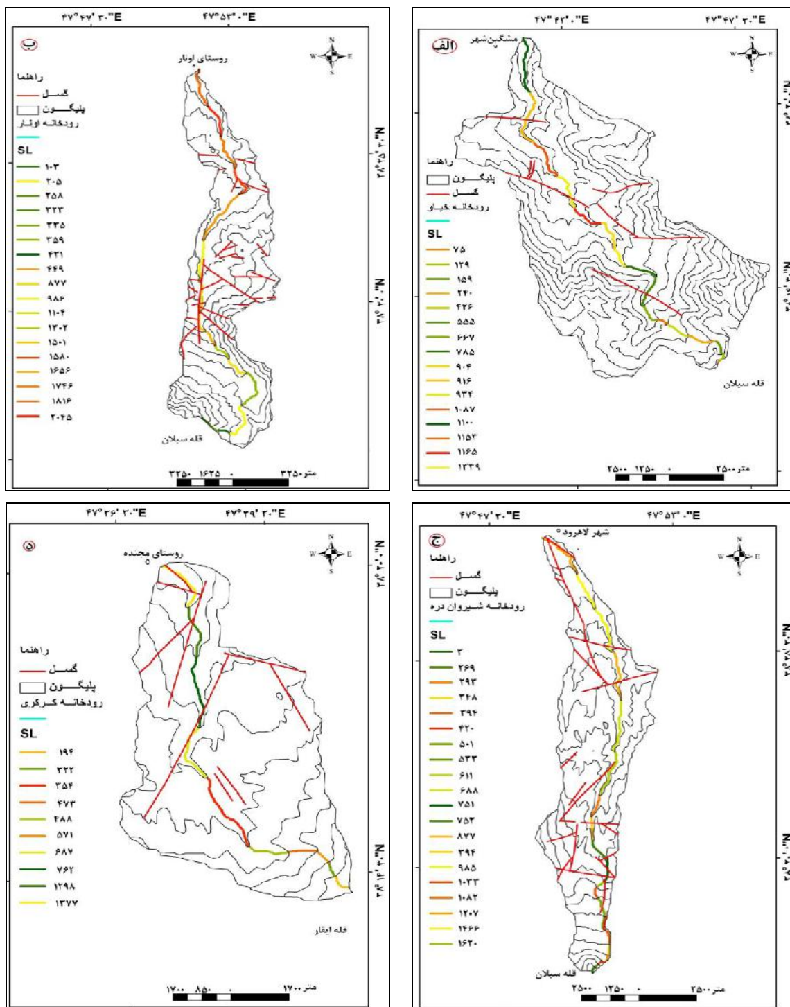
شکل ۳. مقدار شاخص SL در حوضه‌های آبریز؛ الف: خیاو؛ ب: اوانار؛ ج: شیروان درّه و د: کرکری
