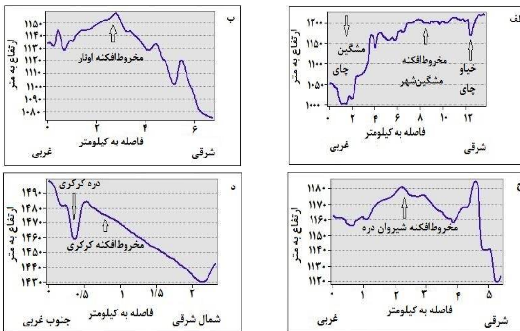
شکل ۴. پروفیل‌های عرضی مخروط‌افکنه‌ها؛ الف: مشگین شهر؛ ب: اونار؛ ج: شیروان دره و د: کرگری
