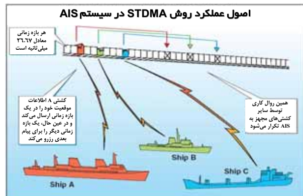
روش تخصیص زمان ارسال اطلاعات برای فرستنده‌های AIS
