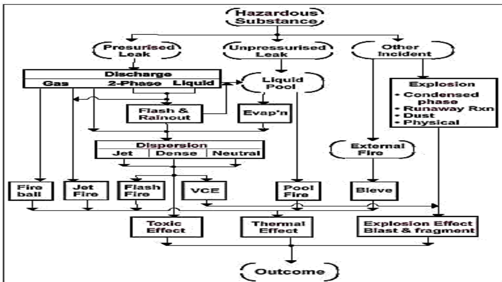
شکل ۱- پیامد ناشی از انتشار، نشتی و رهایش مواد هیدروکربنی
