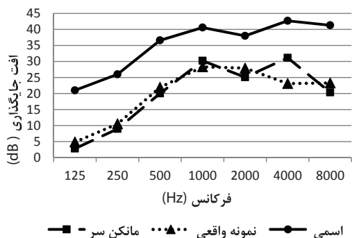
تصویر ۴: مقایسه افت جایگذاری صدای گوشه‌های مدل B در یک اکتاوباند
