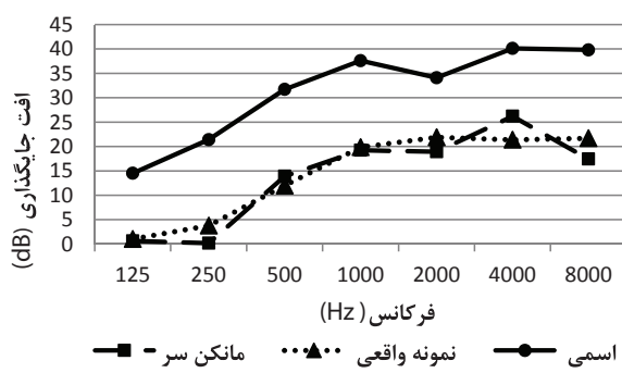
تصویر ۳: مقایسه افت جایگذاری صدای گوشه‌های مدل E در یک اکتاوباند
