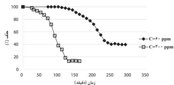
تصویر ۵: حذف فوتوکاتالیستی استتاین (دبی: ۱ lit/min، دما: ۳۲°C، مقدار بستر: gr 2 رطوبت: ۱ ± ۳۵)
