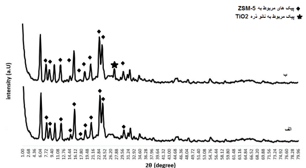
تصویر ۱: الگوی پراش پرتو X، پراش الف مربوط به ZSM-5 و پراش ب مربوط به TiO 2 /ZSM-5 می‌باشد
