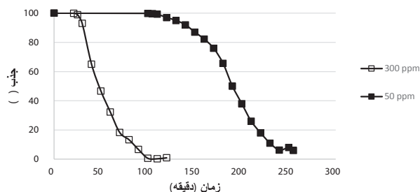
تصویر ۴: بررسی میزان جذب ZSM-5 در دو غلظت ۵۰ و ۳۰۰ پی پی ام (دما: ۳۲°C، مقدار بستر: gr۲، رطوبت: ۱ ± ۳۵، لامپ UV روشن)
