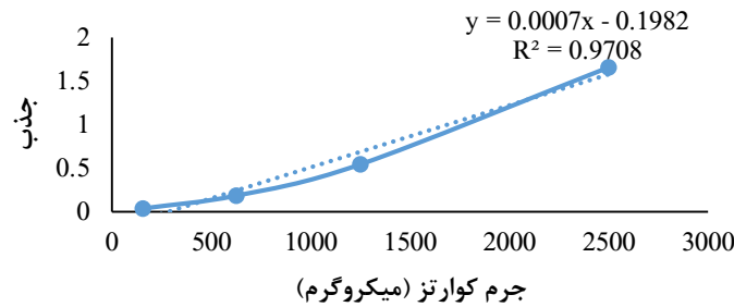
منحنی کالیبراسیون
