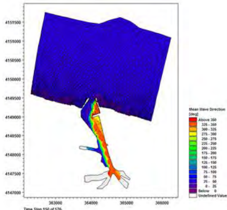
شکل (۶): جهت و ارتفاع مشخصه امواج، قبل و بعد از توسعه موج شکن های بندرانزلی در زمان وزش باد شمال شرقی
