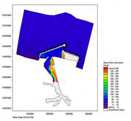
شکل (۷): جهت متوسط امواج، قبل و بعد از توسعه موج شکن های بندرانزلی در زمان وزش باد شمال شرقی
