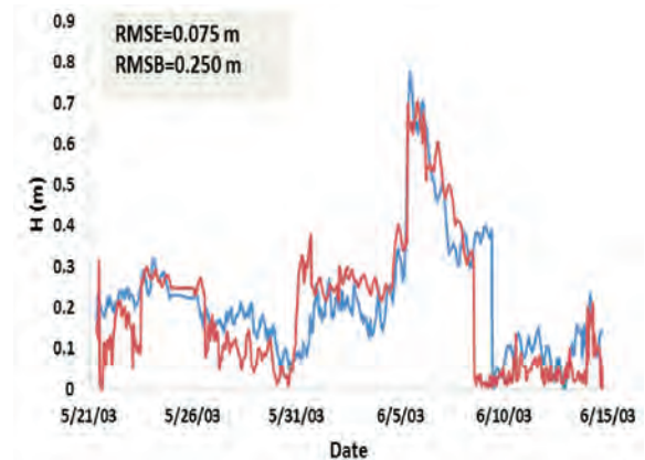
شکل (۲): مقایسه تغییرات ارتفاع موج ثبت‌شده با مقادیر شبیه‌سازی شده توسط مدل در محدوده بندر
