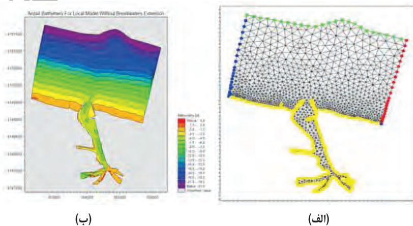
شکل (۵): (الف) شبکه‌بندی و (ب) نقشه عمق‌سنجی محدوده مطالعاتی در مدل محلی بدون توسعه بازوهای موج‌شکن
