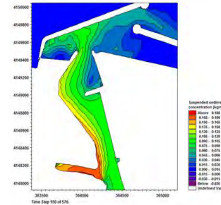
شکل (۹): تغییرات غلظت جریان رسوبات، قبل و بعد از توسعه موج شکن های بندرانزلی در زمان وزش باد شمال شرقی
