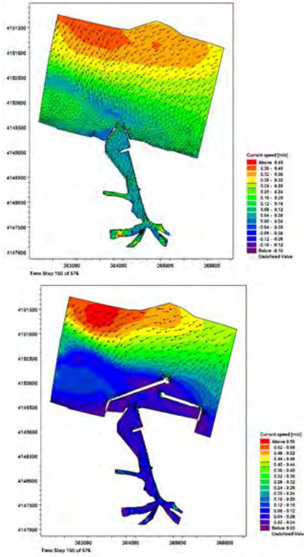
شکل (۸): تغییرات سرعت جریان، قبل و بعد از توسعه موج شکن های بندرانزلی در زمان وزش باد شمال شرقی
