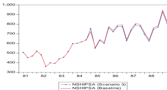
شکل (۴): اثر افزایش ۵ درصدی نرخ ارز بر تابع تقاضای ورود کشتی به بندر شهید رجایی (با در نظر گرفتن هم زمان تأثیر نرخ ارز بر عرضه صادرات غیرنفتی و واردات کل)
