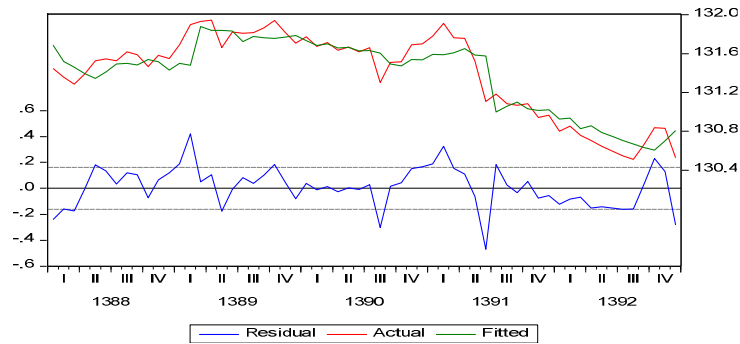
نمودار ۳-۴. نمودار خطی پسماند مدل رگرسیونی سوم
