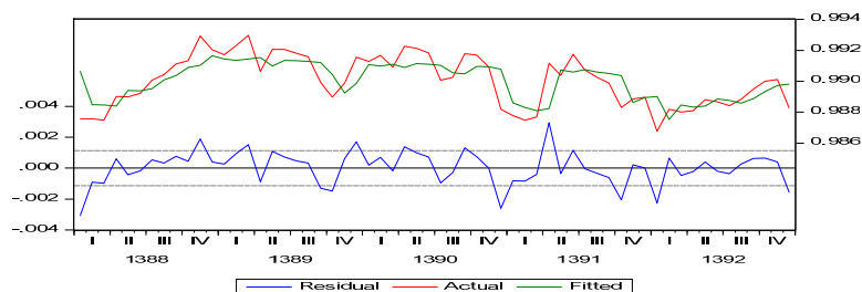
نمودار ۲-۴. نمودار خطی پسماند مدل رگرسیونی دوم
