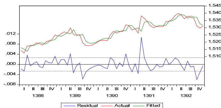
نمودار ۴-۱. نمودار خطی پسماند مدل رگرسیونی اول
