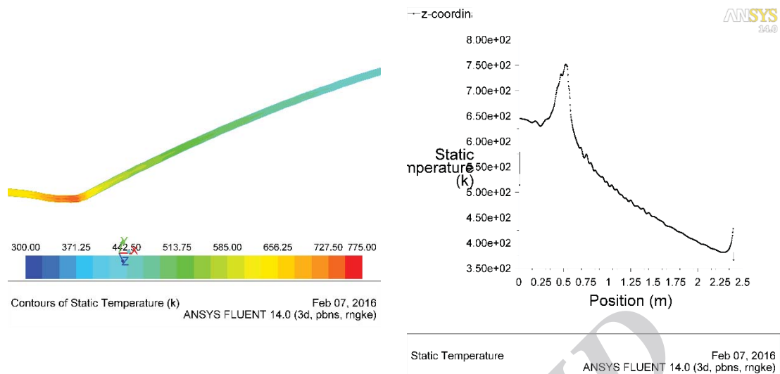
شکل ۱۲- دما روی خط مرکزی صفحه‌ی بین محفظه گاز داغ و سیال خنک کاری
