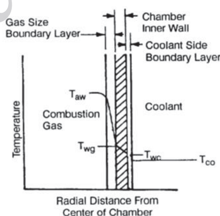
شکل ۱ - شماتیک انتقال حرارت برای خنک کاری بازبایی [۲]
