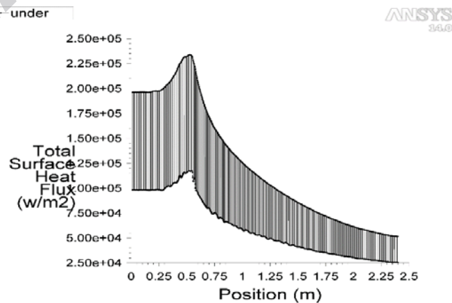
شکل ۹- شار حرارتی اعمال شده روی مرز متصل به منبع گرمایی (نازل پیشرانش
