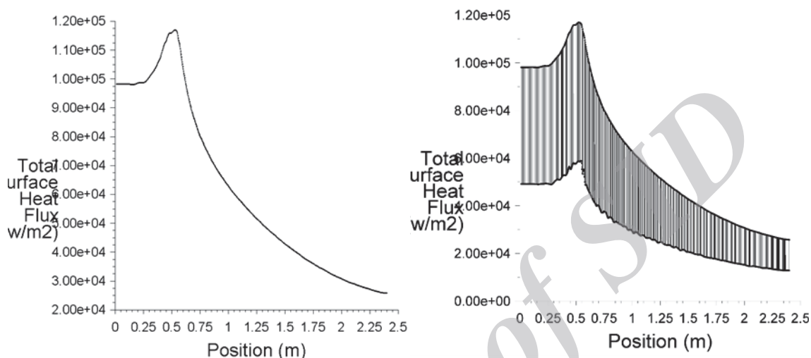
شکل ۶ - پروفیل شار گرمایی اعمال شده روی دیواره
