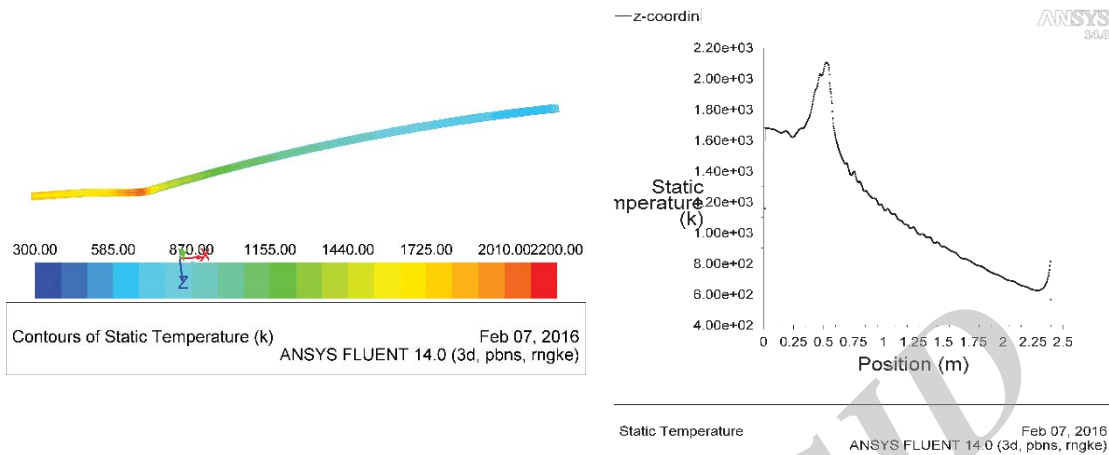
شکل ۱۰- دمای روی خط مرکزی صفحه‌ی بین محفظه گاز داغ و سیال خنک کاری
