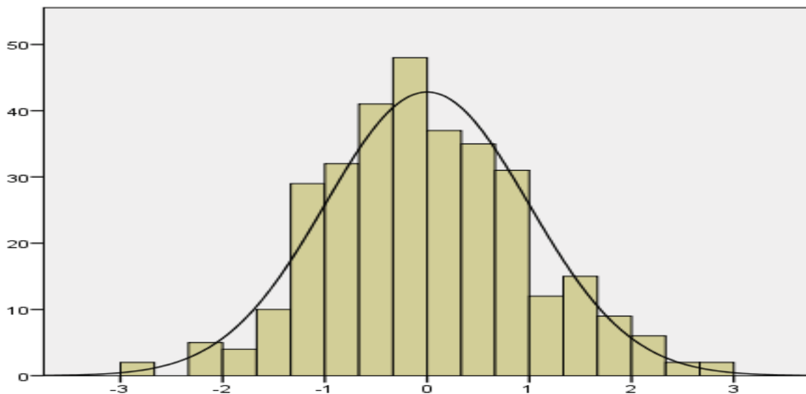
نمودار ۳. هیستوگرام نرمات باقی مانده یادگیری خودراهربر از طریق راهبردهای فراشناختی
