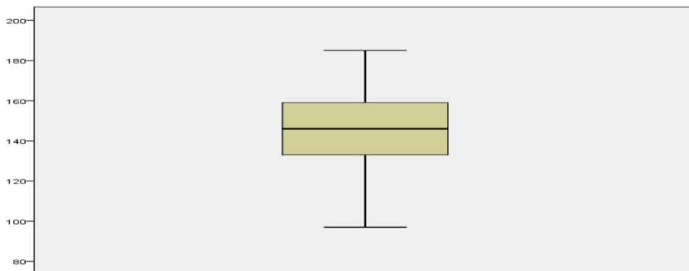
نمودار ۱. نمودار جعبه‌ای نمرات یادگیری خودراهبر دانش‌آموزان برای بررسی وجود داده پرت
