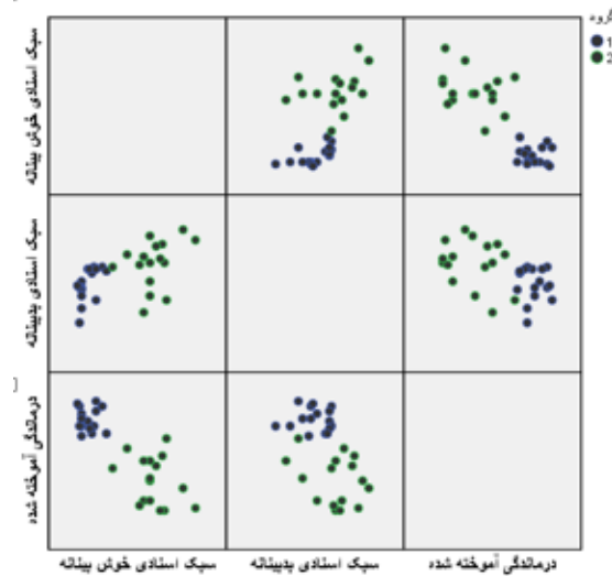
شکل ۱: نمودار پراکنش برای بررسی خطی بودن رابطه بین متغیرها
