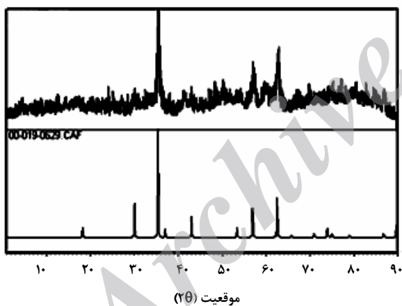
شکل ۲- الگوی پراش XRD نانوذرات مگنتیت سنتز شده در مقایسه با الگوی پراش مرجع مگنتیت
