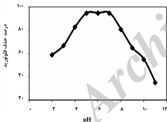
شکل ۵- اثر pH بر حذف فلئوئورید
