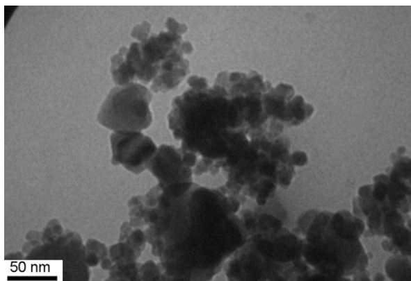
شکل ۳- تصویر TEM نانوجاذب تهیه شده
