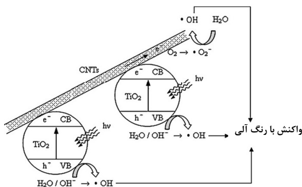
شکل ۱۳- مکانیسم فوتوکاتالیزی (CNT/TiO 2 ) برای
