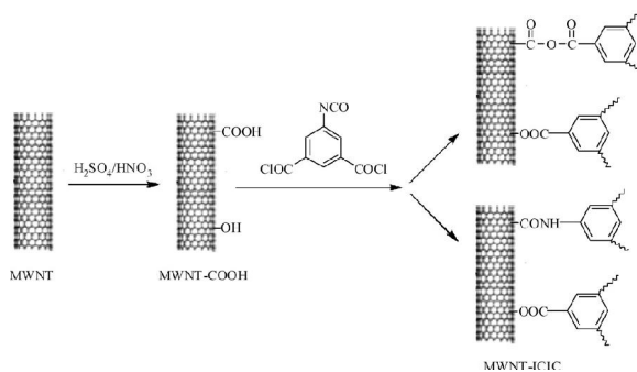
شکل ۸- فرایند اصلاح MWCNT [۲۳]
