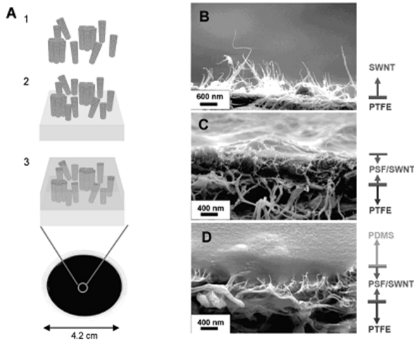
شکل ۱۱- قراردادن CNTها در غشای متخلخل: مرحله ۱: پخش کردن CNT در حلال نتراهیدروفوران، مرحله ۲: صاف کردن محلول نانولوله از غشای تفلونی (شکل B)، مرحله ۳: پوشش سطح غشاء با لایه بسیار (شکل‌های C و D) [۲۵]
