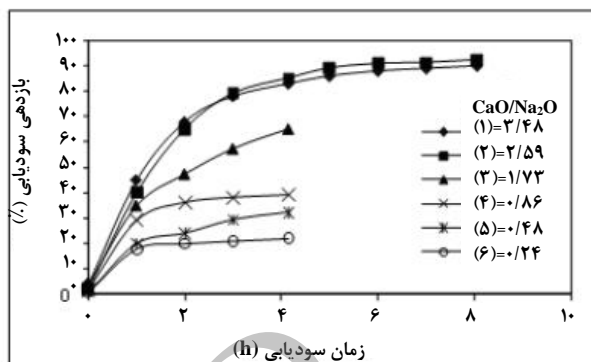
شکل ۲- تأثیر مقادیر مختلف نسبت CaO/Na 2 O در بازدهی سودیابی
