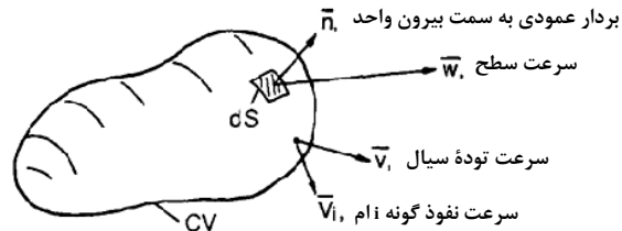
شکل ۱- نمادگذاری حجم کنترل
