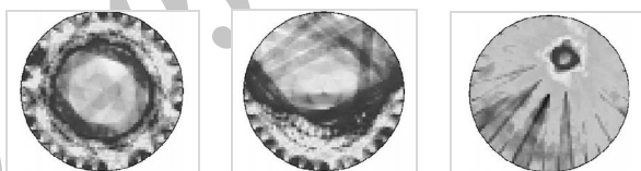
شکل ۹- تصویر بازسازی شده توسط الگوریتم و افکنش خطی (الف) جریان حبابی، (ب) جریان لایه‌ای ۵۵٪، (ج) جریان حلقوی [۱۶]
