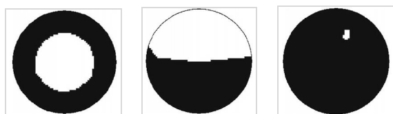
شکل ۱۰- تصویر بازسازی شده توسط الگوریتم بازسازی هیبریدی دوتایی (الف) جریان حبابی، (ب) جریان لایه‌ای ۵۵٪، (ج) جریان حلقوی [۱۶]
