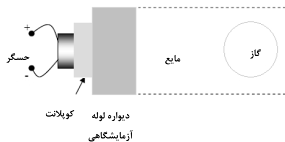
شکل ۲- نمایش نصب حسگر فراصوت روی لوله
